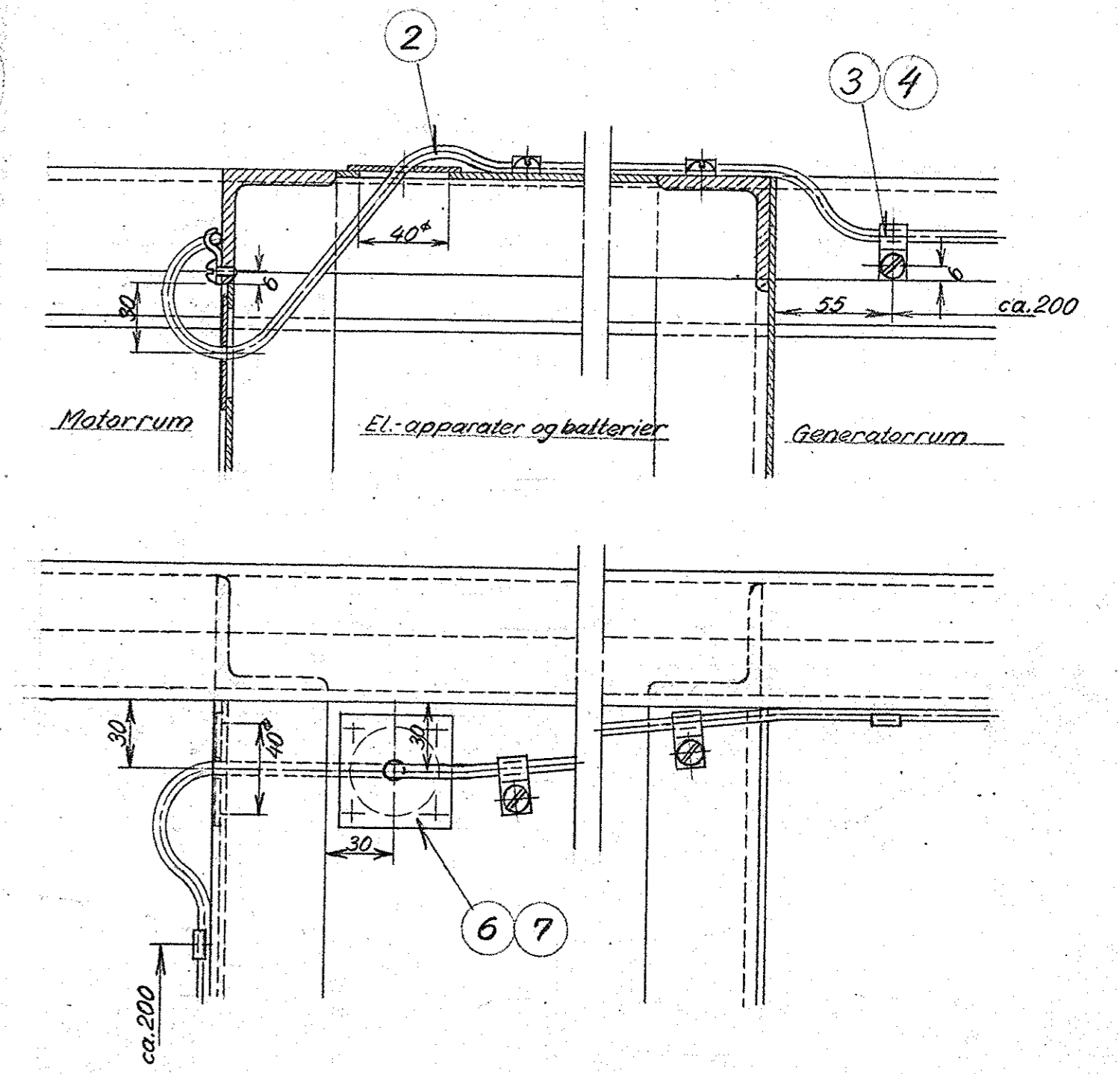
Detail A; 1:2,5
